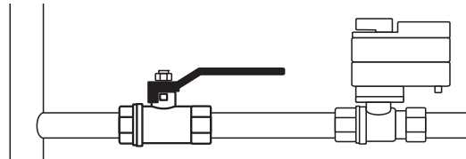
Рис. 2. Схема установки крана шарового с электроприводом.
